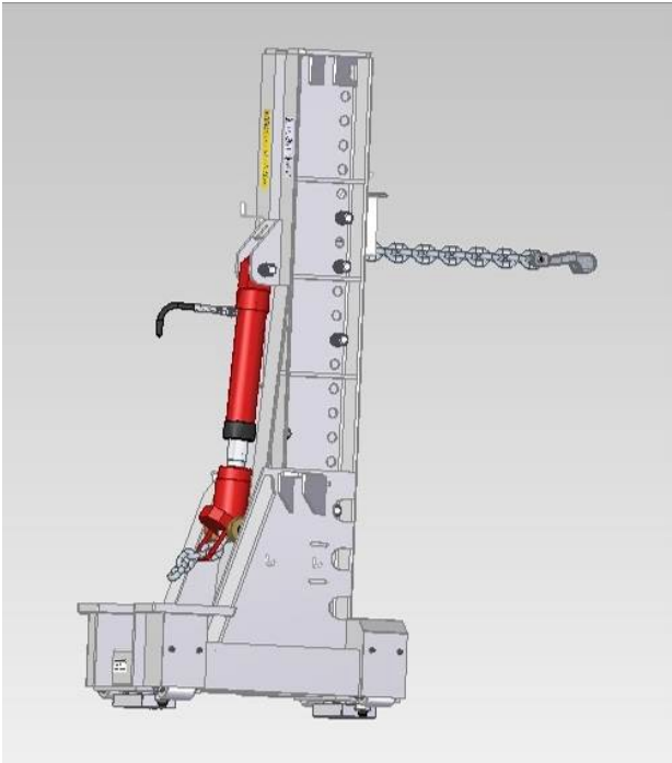
23T solo tiro
